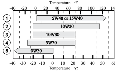
Figura 11: Tabla de viscosidad del aceite del motor
