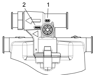
Illustration 14 : Vanne de mélange du carburant
