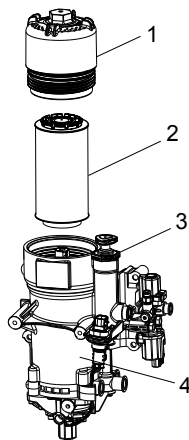
Illustration 13 : Module de filtration du carburant
